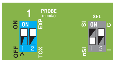
Microinterruttore: Sonda inserita/esclusa
