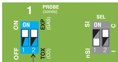
Microinterruttore: Sonda rilevazione gas esplosivo o tossico
