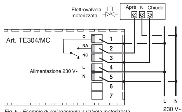
Fig. 5 - Esempio di collegamento a valvola motorizzata
