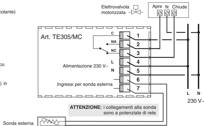
Fig. 6 - Esempio di collegamento a valvola motorizzata e sonda esterna
